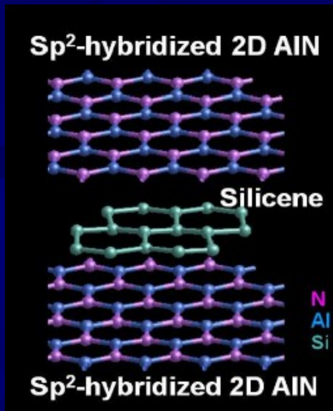
Fig. Silicene – med dvema plastema alum. nitrida AlN
